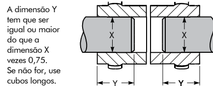
Engrenamento duplo
